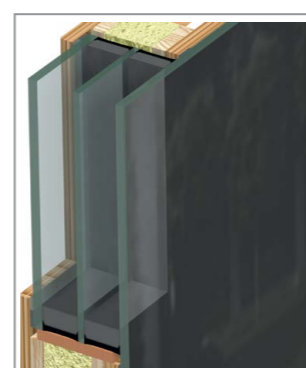
3-fach Verglasung mit Email Außen Klaglas oder Parsol grau mit email schwarz / mittig Klarglas oder Satinato weiß / innen Klarglas Holz & Holz-Alu Serie VETRO
