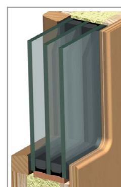
3-fach Verglasung Oramentglas mittig / außen und innen Klarglas Holz
